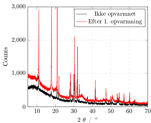
(a) 1:6 XRD-data
