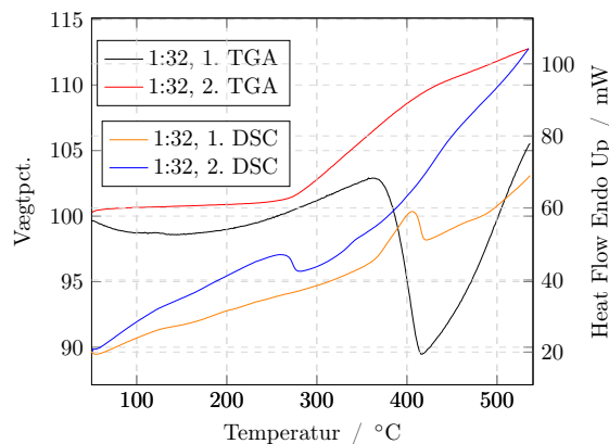
(b) 1:32 TGA/DSC-data
