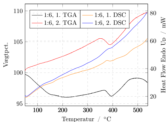
(a) 1:6 TGA/DSC-data
