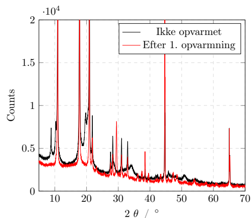
(b) 1:32 XRD-data
